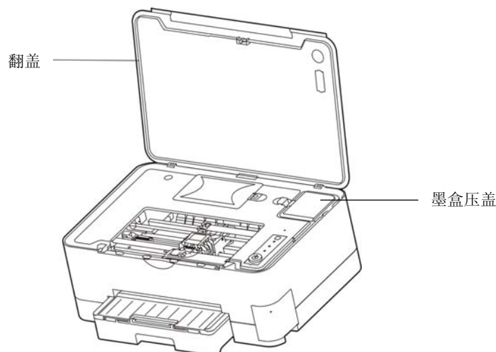
图 A-1 打开翻盖并取出墨盒压盖
