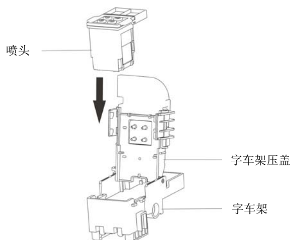
图 A-7 安装喷墨头
