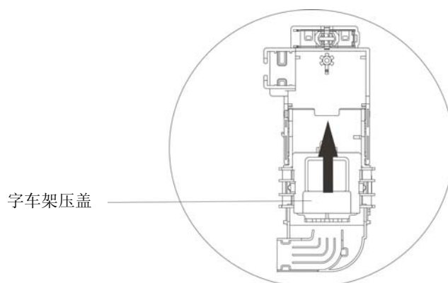
图 A-8 锁紧字车架压盖
