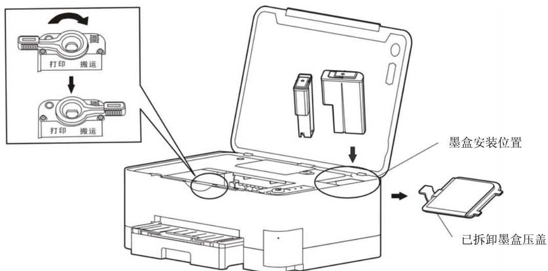
图 2-11 安装墨盒
